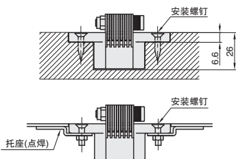
安装图
