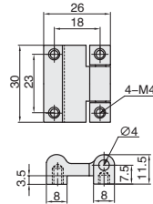
HGPZRK 螺孔型
