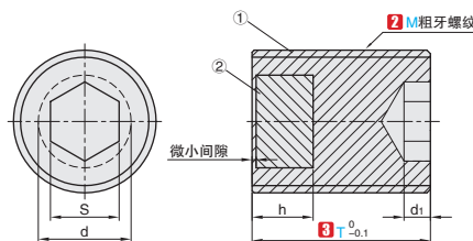
MTBULL 内六角孔型
