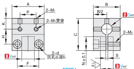
FCSBJ FCSEJ FCSNJ FCSCJ FCSAJ 异径正交带安装孔型
