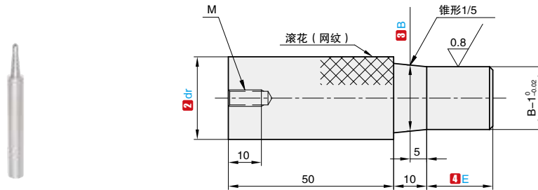
无台阶锥形 dr=8-25
