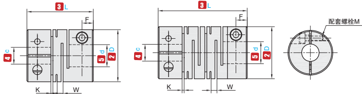
短型(例: CPCIG-16-16)
