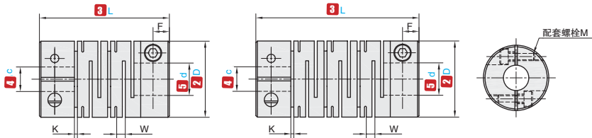
短型(例: CPCIG-40-50)
