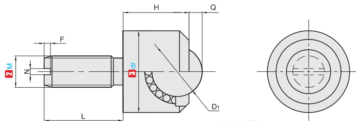
JCAS/JCBS 圆头外螺纹杆锥型
