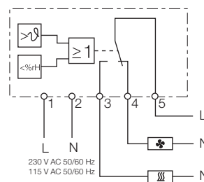
Diagrama eléctrico
