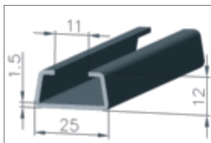
Universelle Doppel- und Gegenwannen
