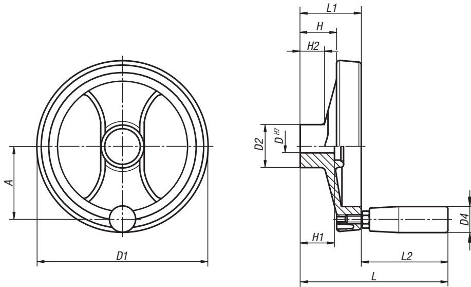
Passfedernut nach DIN 6885-1
