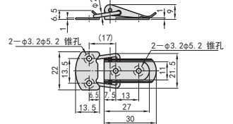
推荐安装孔间距
