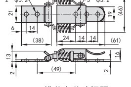
推荐安装孔间距
