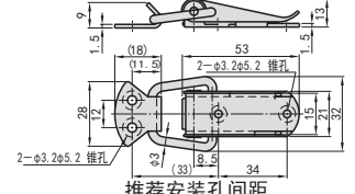
推荐安装孔间距
