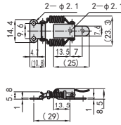
推荐安装孔间距
