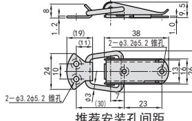
推荐安装孔间距
