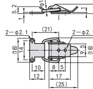
推荐安装孔间距
