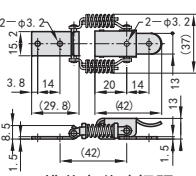
推荐安装孔间距
