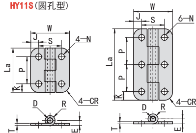
HY11S (圆孔型)
