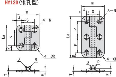
HY12S (锥孔型)
