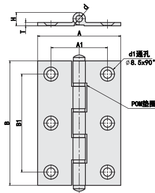
■ 6孔安装
