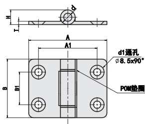
■ 4孔安装
