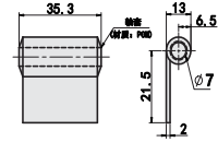
活动连接件
