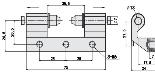
活动连接件
